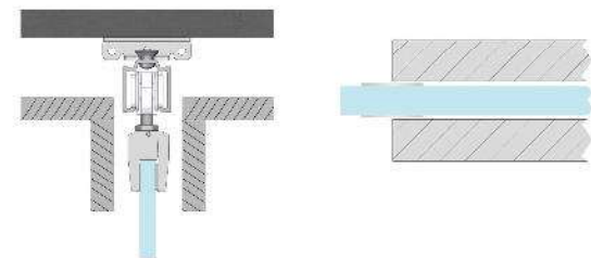
Deckenbündige Montage
