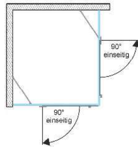
TY ED 5052
