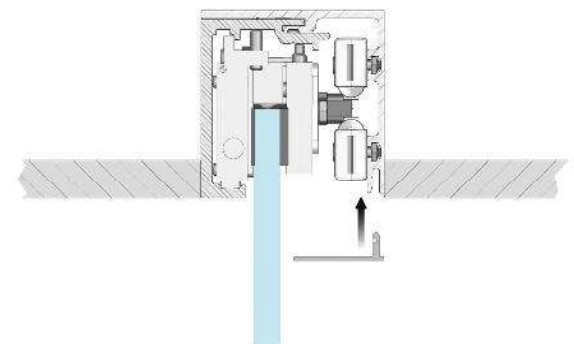
Deckenbündige Montage
